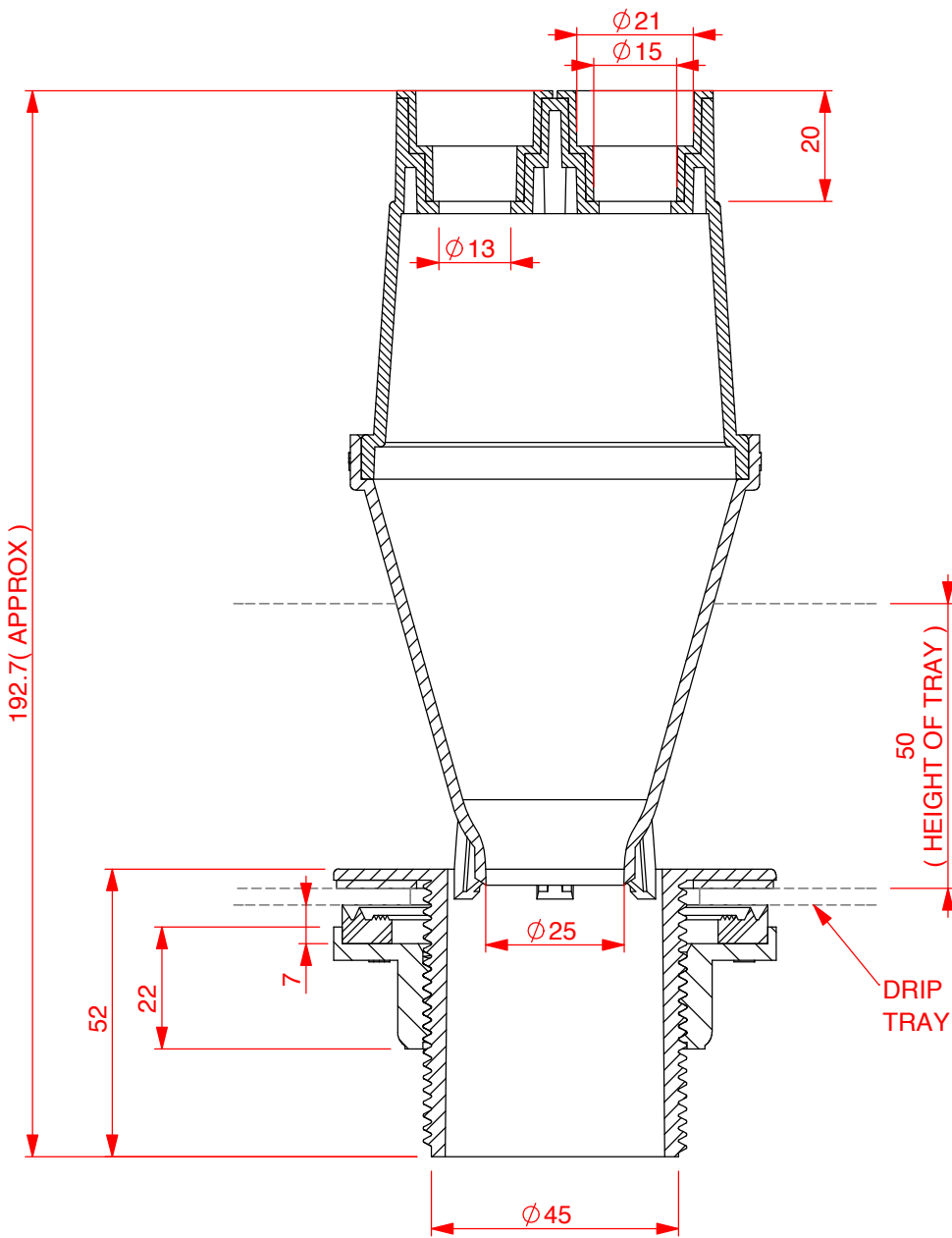
SECTION A-A
